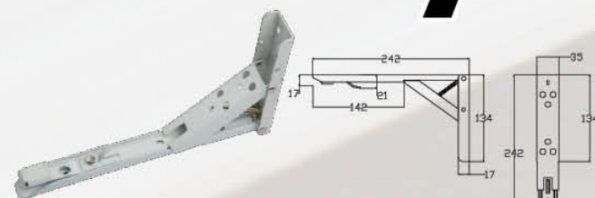
— STB101 — 材质: 铁 — Material: Iron
