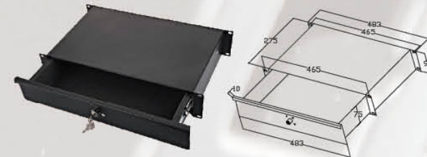
RAG101 表面处理: 喷涂 Finish: Powder Coated 材质: 铁 Material: Iron 重量: 5.66kg Weight: 5.66kg
