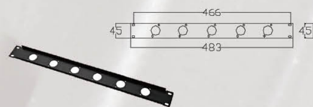
RAB403 表面处理: 喷涂 Finish: Powder Coated 材质: 铁 Material: Iron 重量: 250克 Weight: 250g
