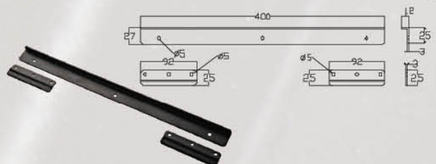
RAD101 表面处理: 喷涂 Finish: Powder Coated 材质: 铁 Material: Iron 重量: 303克 Weight: 303g
