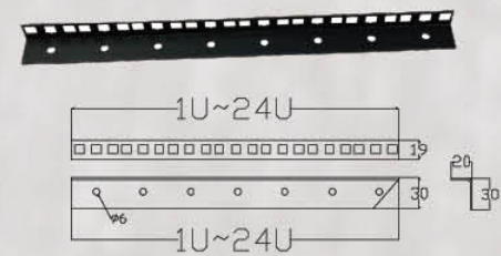
— RAA301 — 材质: 铁 — Material: Iron — 表面处理: 喷涂 — Finish: Powder Coated
