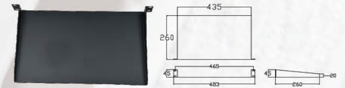
RAF102 表面处理: 喷涂 Finish: Powder Coated 材质: 铁 Material: Iron 重量: 1.415kg Weight: 1.415kg
