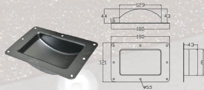
— DIA201 — 材质: 铁 — Material: Iron
