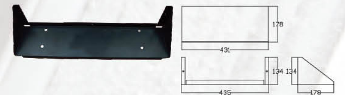
RAF301 表面处理: 喷涂 Finish: Powder Coated 材质: 铁 Material: Iron 重量: 1.034kg Weight: 1.034kg
