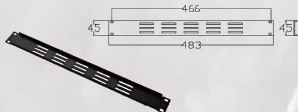
RAB402 表面处理: 喷涂 Finish: Powder Coated 材质: 铁 Material: Iron 重量: 260克 Weight: 260g
