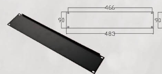
— RAB302 — 材质: 铁 — Material: Iron — 表面处理: 喷涂 — Finish: Powder Coated — 重量: 439克 — Weight: 439g
