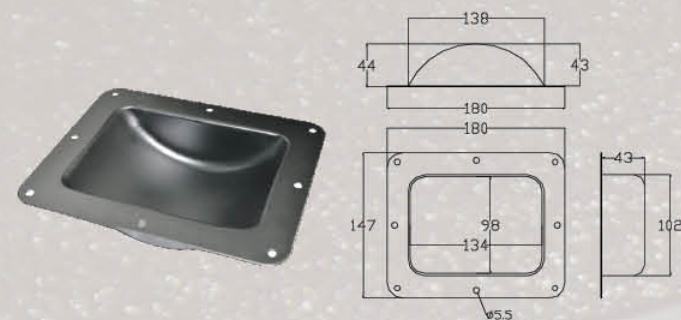
— DIA101 — 材质: 铁 — Material: Iron
