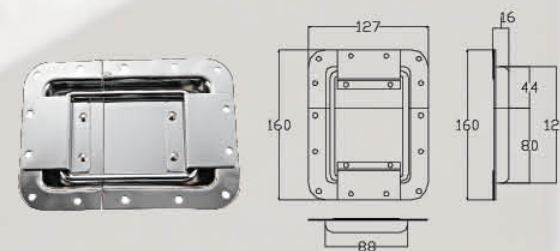
STA201 材质: 铁 Material: Iron 表面处理: 镀铬 Finish: Chrome Plated 重量: 452克 Weight: 452g
