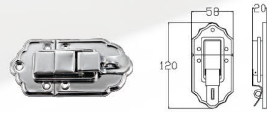
— LOB101 — 材质: 铁 — Material: Iron
