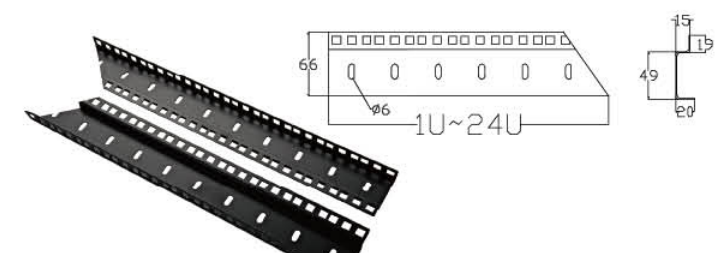
— RAA102 — 材质: 铁 — Material: Iron
