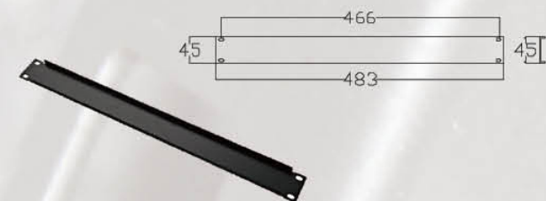
RAB401 表面处理: 喷涂 Finish: Powder Coated 材质: 铁 Material: Iron 重量: 274克 Weight: 274g
