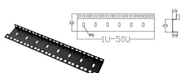
— RAA101 — 材质: 铁 — Material: Iron
