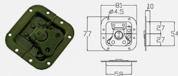
— LOA303 — 材质: 铁 — Material: Iron
