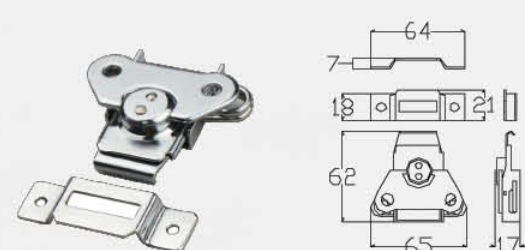
— LOA401 — 材质: 铁 — Material: Iron
