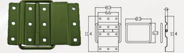
HIC202 材质: 铁 Material: Iron 表面处理: 喷涂 Finish: Powder Coated 重量: 149克 Weight: 149g
