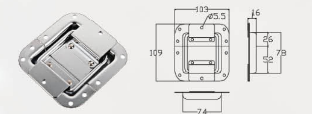
STA301 材质: 铁 Material: Iron 表面处理: 镀铬 Finish: Chrome Plated 重量: 235.5克 Weight: 235.5g
