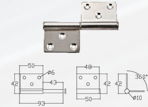
HIA101 材质: 不锈钢 Material: Stainless Steel 表面处理: 拉丝 Finish: Brushed 重量: 106克 Weight: 106g
