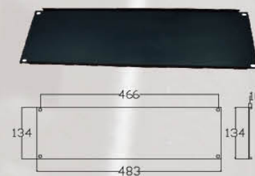
— RAB201 — 材质: 铁 — Material: Iron — 表面处理: 喷涂 — Finish: Powder Coated — 重量: 691.5克 — Weight: 691.5g
