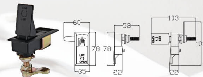
— LOC101 — 材质: 铁 — Material: Iron
