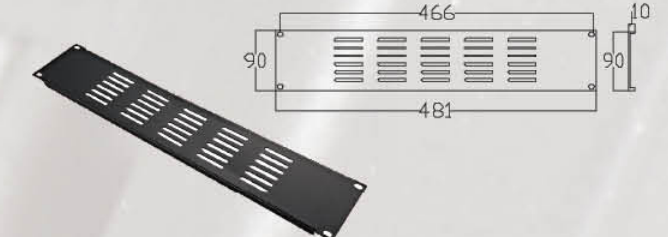
— RAB303 — 材质: 铁 — Material: Iron — 表面处理: 喷涂 — Finish: Powder Coated — 重量: 436克 — Weight: 436g
