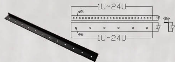
— RAA401 — 材质: 铁 — Material: Iron — 表面处理: 喷涂 — Finish: Powder Coated
