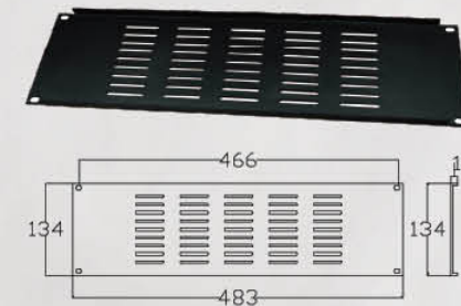
— RAB202 — 材质: 铁 — Material: Iron — 表面处理: 喷涂 — Finish: Powder Coated — 重量: 633克 — Weight: 633g
