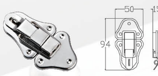
— LOB301 — 材质: 铁 — Material: Iron
