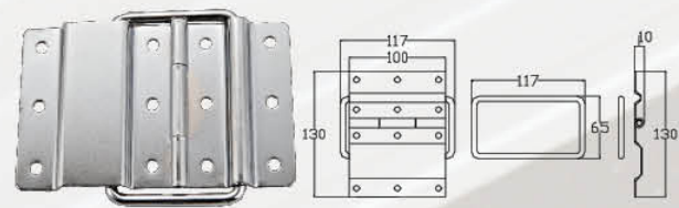
HIC101 材质: 铁 Material: Iron 表面处理: 镀铬 Finish: Chrome Plated 重量: 253克 Weight: 253g
