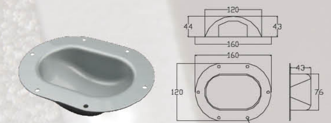
— DIB101 — 材质: 铁 — Material: Iron
