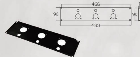
— RAB204 — 材质: 铁 — Material: Iron — 表面处理: 喷涂 — Finish: Powder Coated — 重量: 616.5克 — Weight: 616.5g
