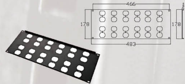
— RAB102 — 材质: 铁 — Material: Iron — 表面处理: 喷涂 — Finish: Powder Coated — 重量: 853.5克 — Weight: 853.5g
