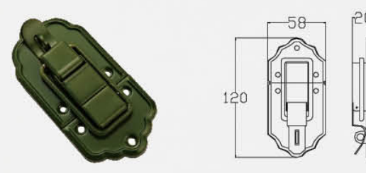
— LOB102 — 材质: 铁 — Material: Iron
