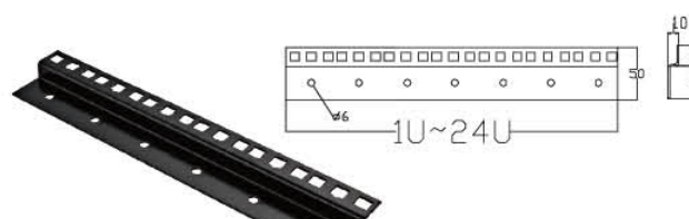
— RAA201 — 材质: 铁 — Material: Iron
