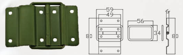
HIC302 材质: 铁 Material: Iron 表面处理: 喷涂 Finish: Powder Coated 重量: 51克 Weight: 51g
