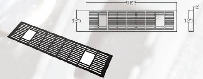
RAE102 表面处理: 喷涂 Finish: Powder Coated 材质: 铁 Material: Iron 重量: 295.5克 Weight: 295.5g
