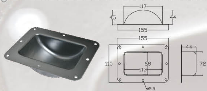
— DIA301 — 材质: 铁 — Material: Iron
