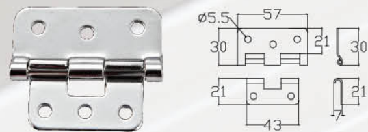
HIB101 材质: 铁 Material: Iron 表面处理: 镀铬 Finish: Chrome Plated 重量: 38克 Weight: 38g
