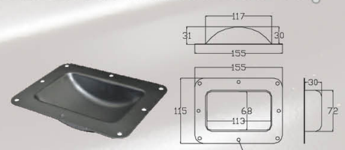
— DIA402 — 材质: 铁 — Material: Iron
