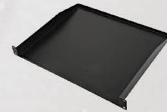
RAF101 表面处理: 喷涂 Finish: Powder Coated 材质: 铁 Material: Iron 重量: 1.48kg Weight: 1.48kg
