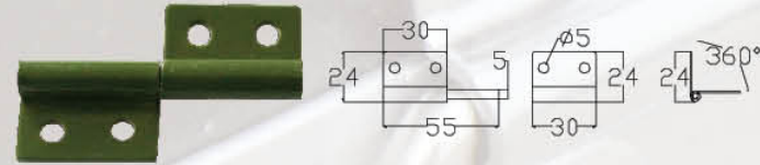
HIA203 材质: 铁 Material: Iron 表面处理: 喷涂 Finish: Powder Coated 重量: 34克 Weight: 34g
