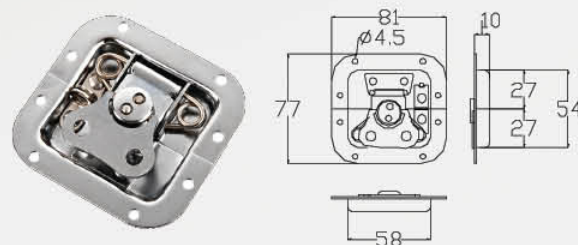
— LOA302 — 材质: 铁 — Material: Iron
