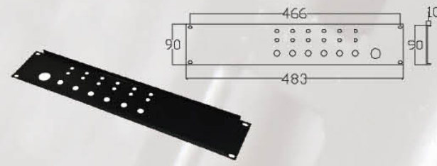
RAB307 表面处理: 喷涂 Finish: Powder Coated 材质: 铁 Material: Iron 重量: 461克 Weight: 461g
