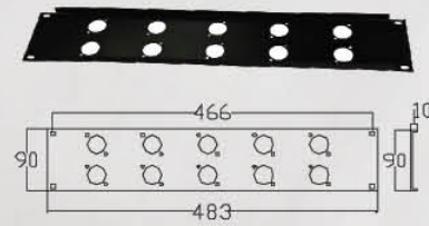
RAB306 表面处理: 喷涂 Finish: Powder Coated 材质: 铁 Material: Iron 重量: 420克 Weight: 420g
