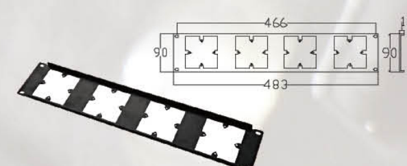
— RAB304 — 材质: 铁 — Material: Iron — 表面处理: 喷涂 — Finish: Powder Coated — 重量: 310克 — Weight: 310g
