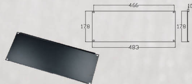
— RAB101 — 材质: 铁 — Material: Iron — 表面处理: 喷涂 — Finish: Powder Coated — 重量: 1043克 — Weight: 1043g
