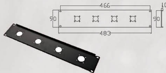
RAB308 表面处理: 喷涂 Finish: Powder Coated 材质: 铁 Material: Iron 重量: 545克 Weight: 545g
