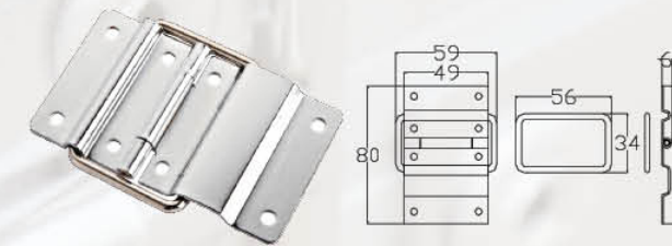
HIC301 材质: 铁 Material: Iron 表面处理: 镀铬 Finish: Chrome Plated 重量: 50.5克 Weight: 50.5g
