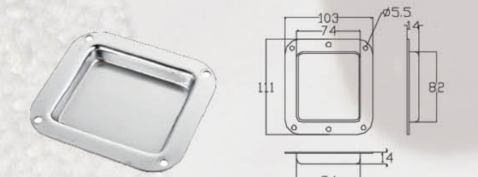
— DID101 — 材质: 铁 — Material: Iron
