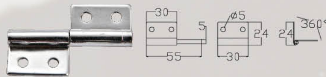
HIA201 材质: 铁 Material: Iron 表面处理: 镀铬 Finish: Chrome Plated 重量: 33.5克 Weight: 33.5g
