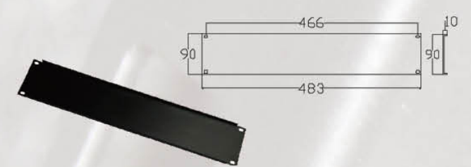
— RAB301 — 材质: 铁 — Material: Iron — 表面处理: 喷涂 — Finish: Powder Coated — 重量: 478.5克 — Weight: 478.5g
