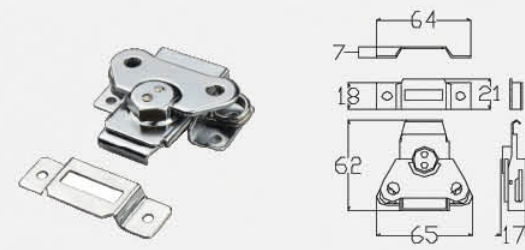
— LOA402 — 材质: 铁 — Material: Iron
